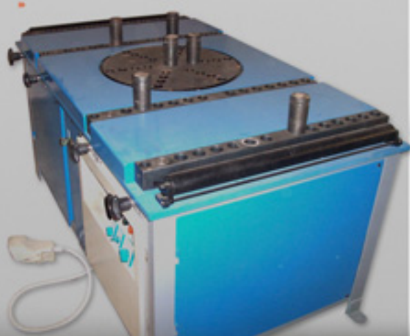
GBT-50 Cintreuse
